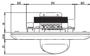
Dimensions LM1-VC12L
