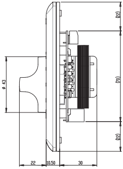
Dimensions LM1-VC12P
