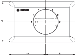
Dimensions LM1-VC12P
